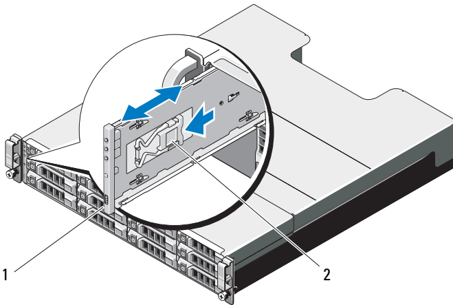
Ilustración 15-13. Extracción e instalación del panel de control de PowerVault MD3200
