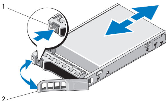
Ilustración 15-4. Extracción e instalación de una unidad de disco duro
