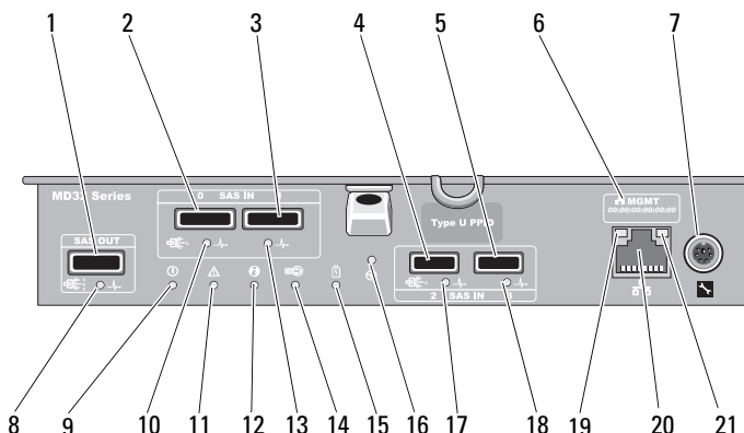
Ilustración 3-1. Módulo de la controladora RAID SAS serie MD3200
