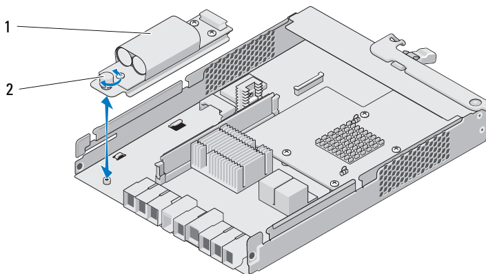
Ilustración 15-10. Extracción e instalación de la unidad de la batería de reserva del módulo de la controladora RAID
