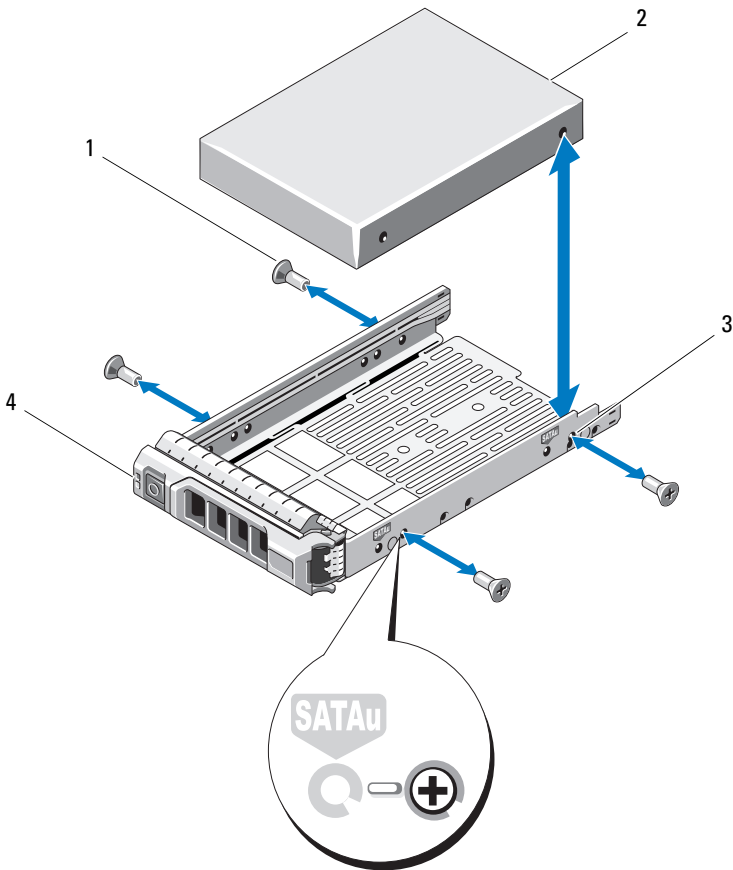
Ilustración 15-5. Extracción e instalación de una unidad de disco duro en un portaunidades de disco duro de 3,5 pulgadas
