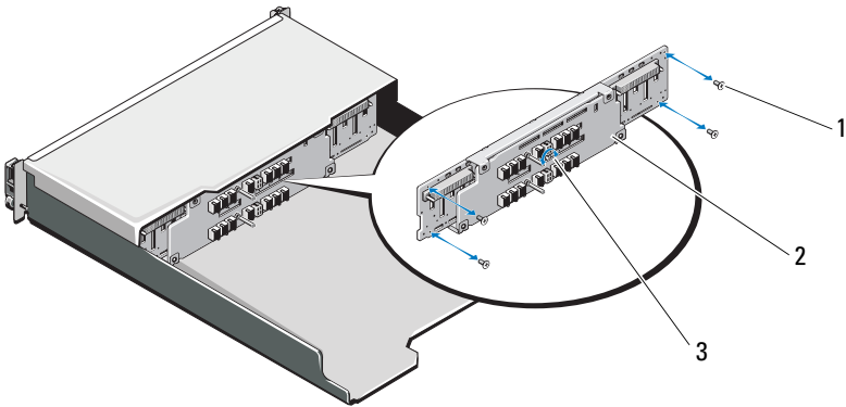
Ilustración 15-17. Extracción e instalación del plano posterior de PowerVault MD3220
