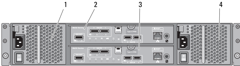
Ilustración 2-4. Indicadores y funciones del panel posterior: Dell PowerVault serie MD3200
