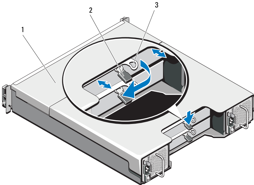
Ilustración 15-8. Extracción e instalación de un módulo de controladora RAID
