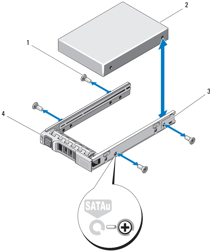
Ilustración 15-6. Extracción e instalación de una unidad de disco duro en un portaunderes de disco duro de 2,5 pulgadas
