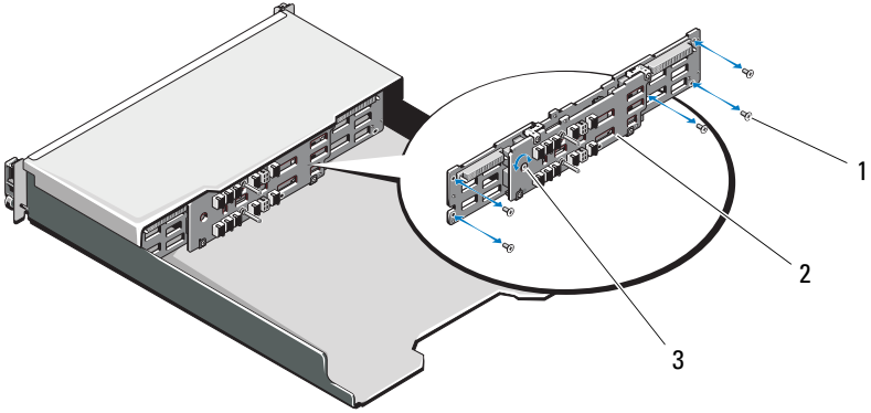
Ilustración 15-16. Extracción e instalación del plano posterior de PowerVault MD3200
