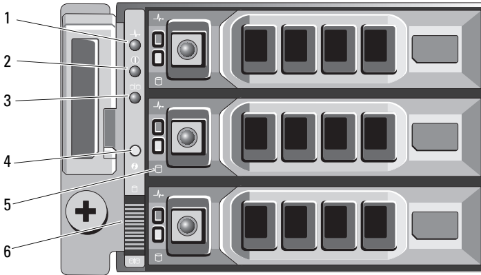
Ilustración 2-2. Indicadores y funciones del panel frontal: Dell PowerVault MD3200
