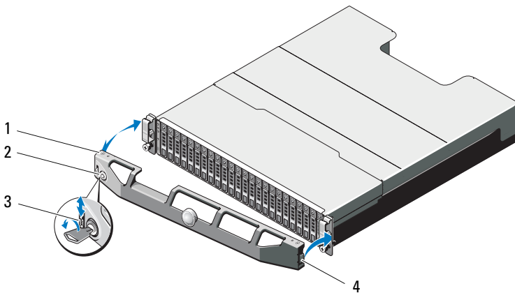
Ilustración 15-1. Extracción e instalación del bisel anterior
