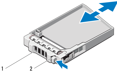
Ilustración 15-3. Extracción e instalación de una unidad de disco duro de relleno de 2,5 pulgadas (solo MD3220).
