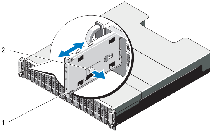
Ilustración 15-14. Extracción e instalación del panel de control de PowerVault MD3220
