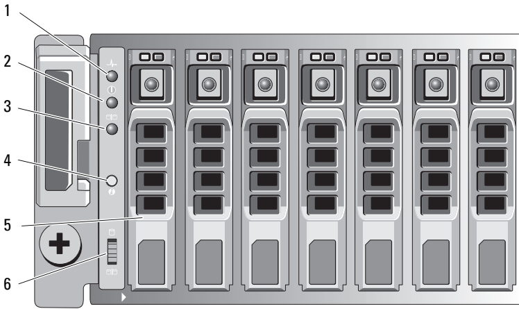
Ilustración 2-2. Indicadores y funciones del panel frontal: Dell PowerVault MD3200
