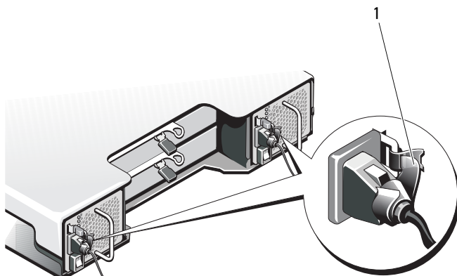
Ilustración 15-12. Fijación del cable de alimentación
